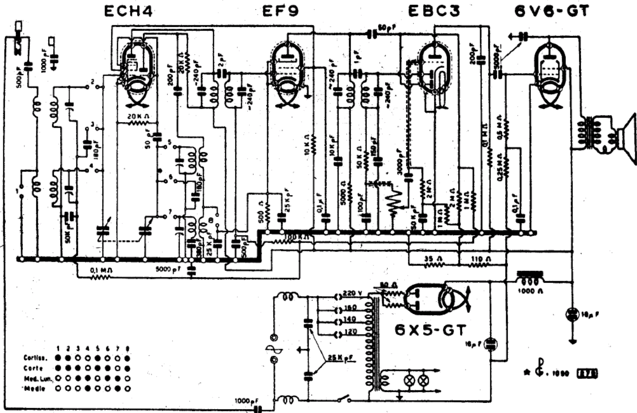
Lo schema elettrico del Phonola 573
